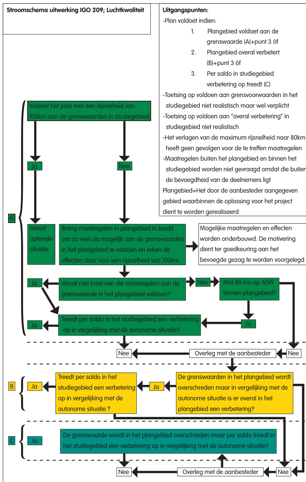
Figuur 3.1 Stroomschema
