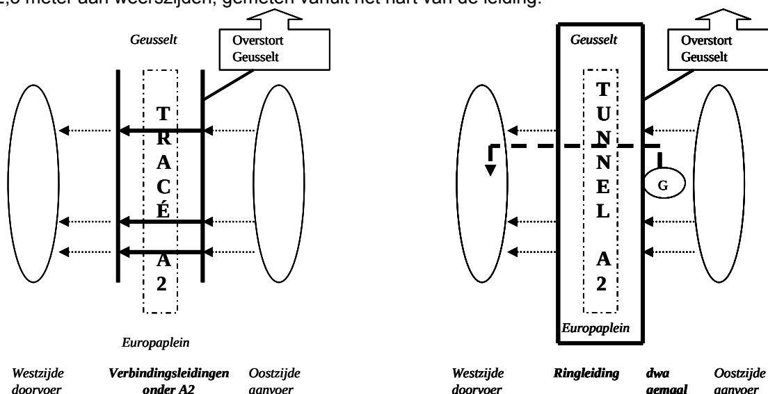
Principeschets van huidige (verbindingsleidingen) en toekomstige (ringleiding) rioleringssituatie
